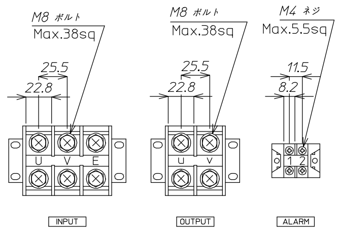
端子台詳細
