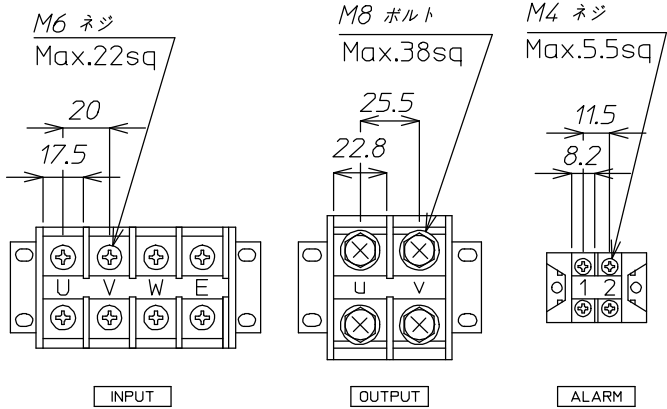
端子台詳細
