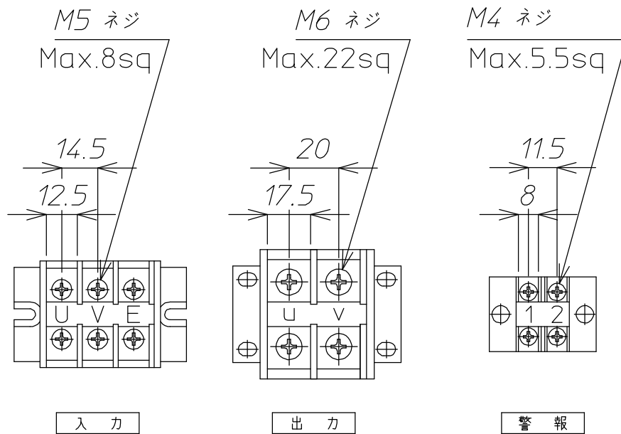
端子台詳細
