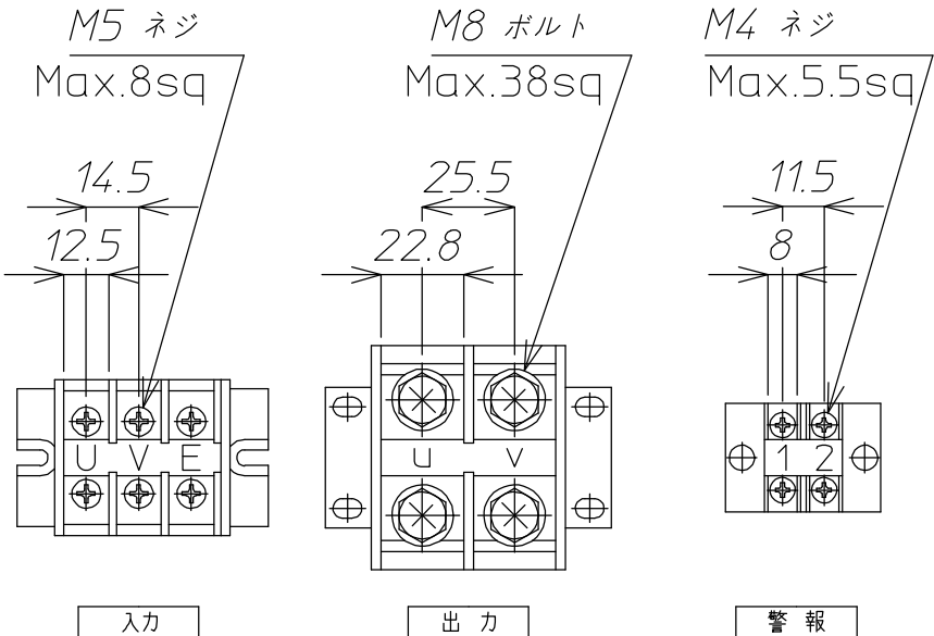
端子台詳細図
