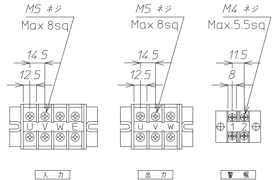
端子台詳細
