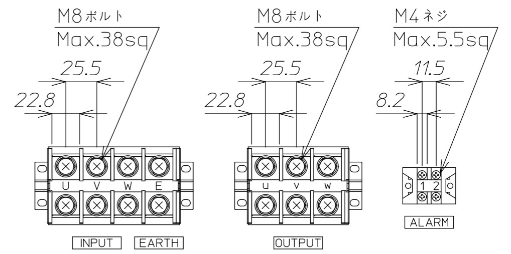
端子詳細図
