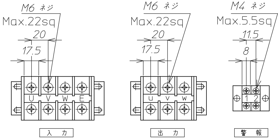
端子台詳細
