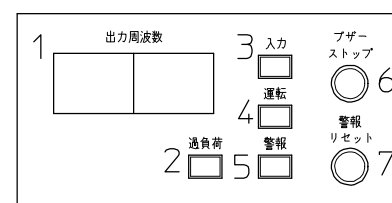
パネル部詳細( 盤面)
