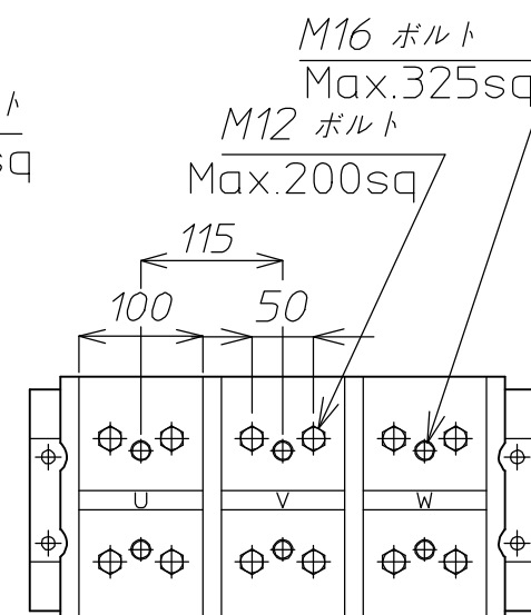
端子台詳細
