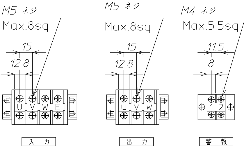
端子台詳細
