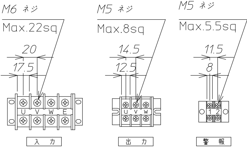
端子台詳細
