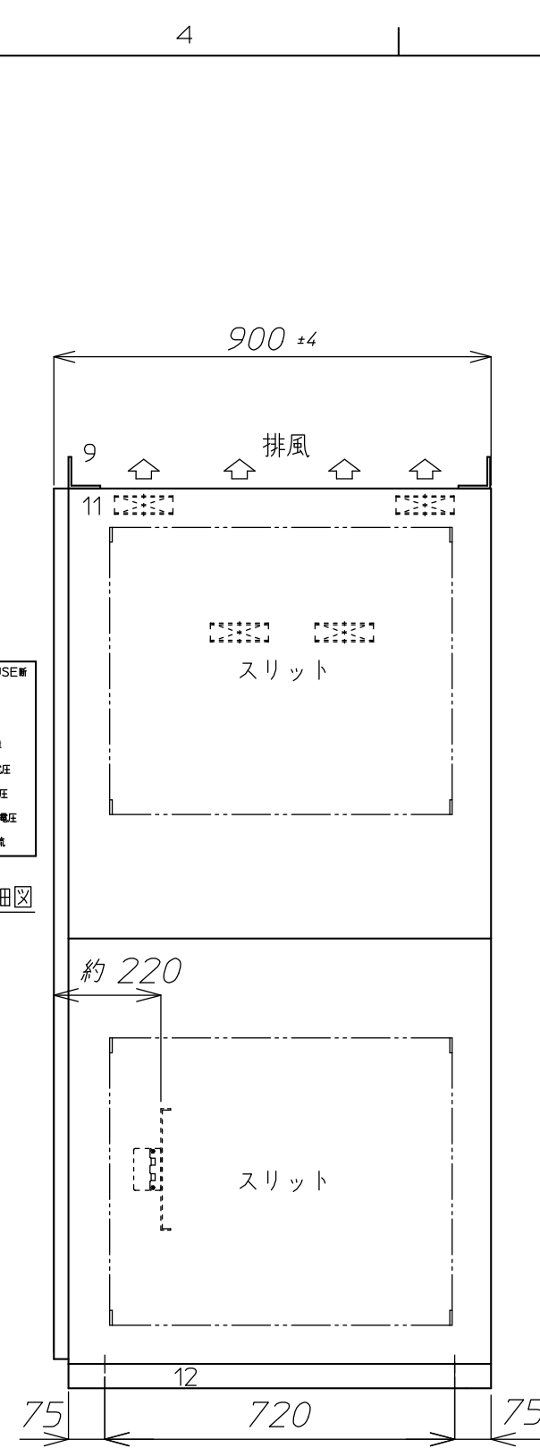
右側面図
