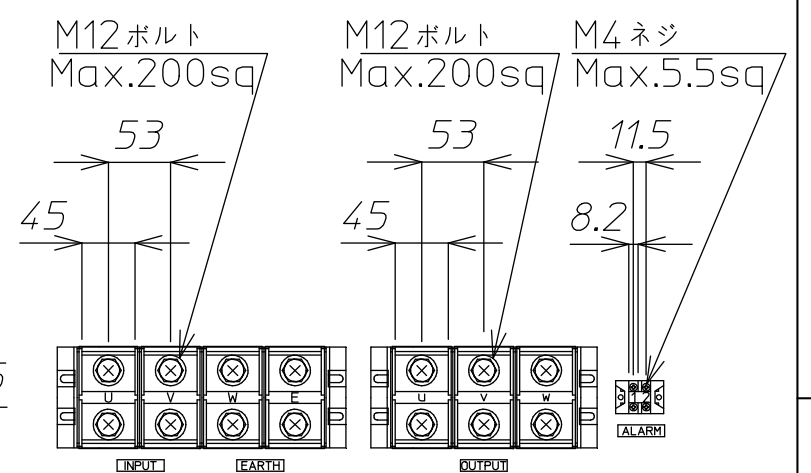
端子詳細図
