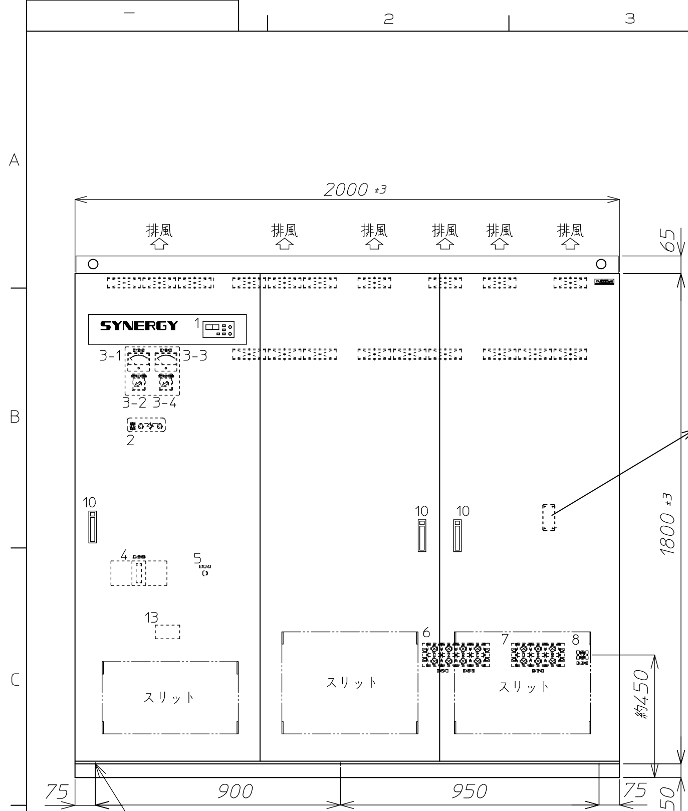
正面図
