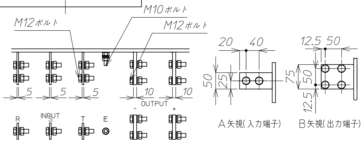
端子板詳細図
