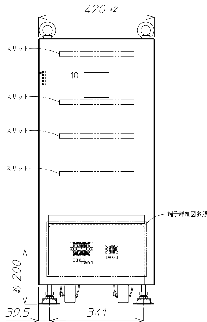
右側面図
